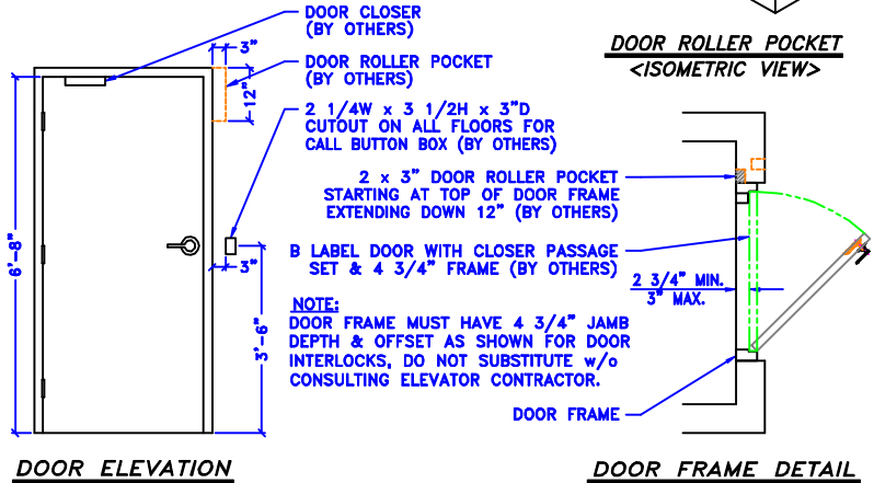
DOOR FRAME DETAIL
