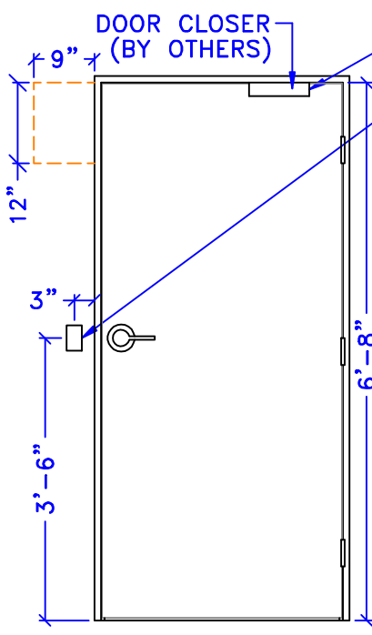
DOOR ELEVATION
