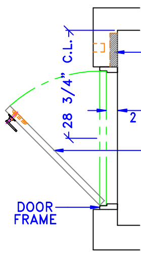
DOOR FRAME DETAIL
